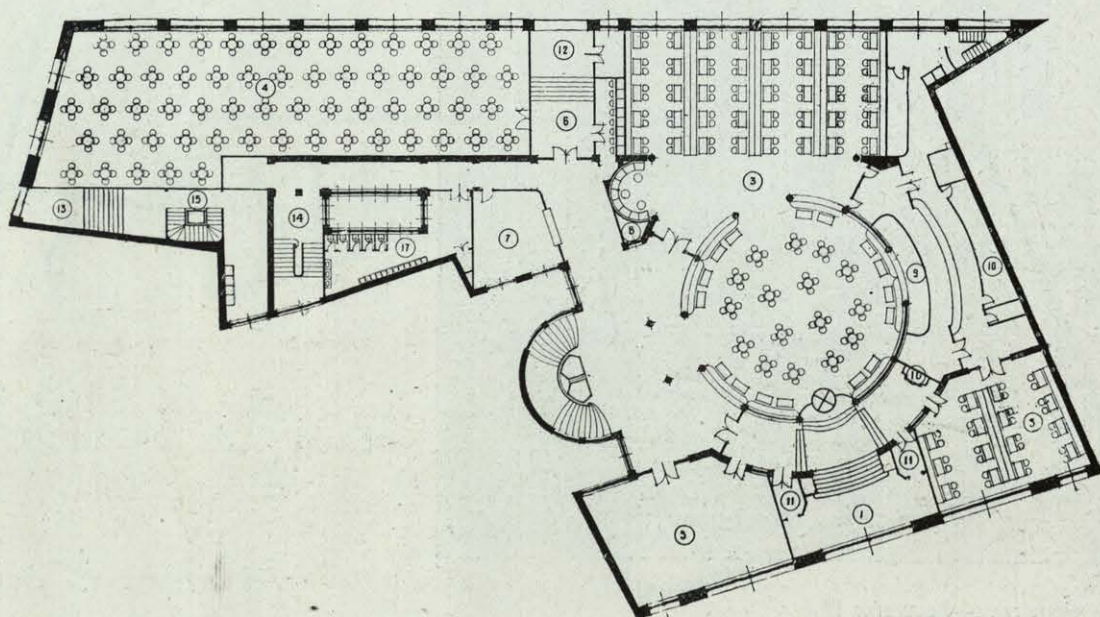
PLANTA BAJA.—SOLUCIÓN D.
