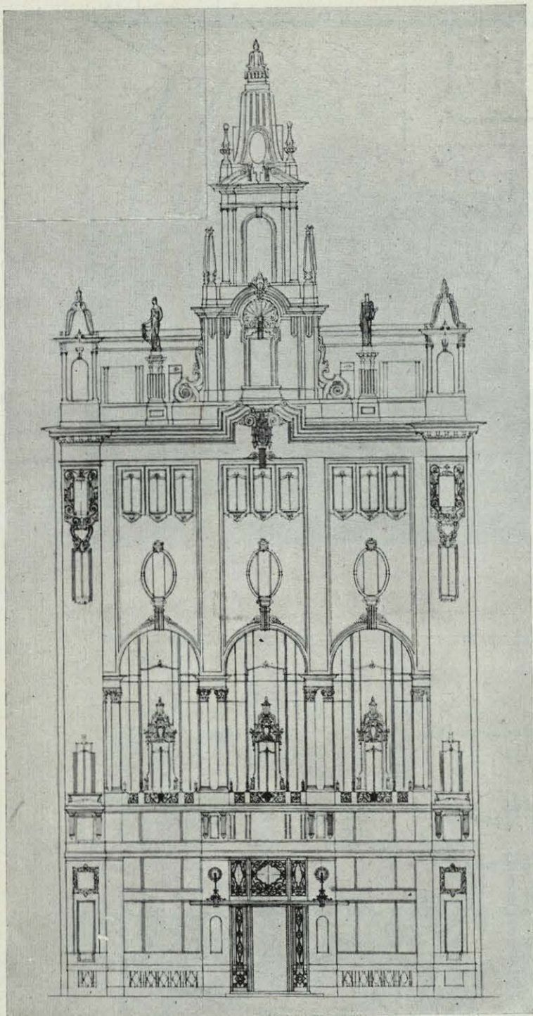
FACHADA PRINCIPAL.—SOLUCIÓN D.
