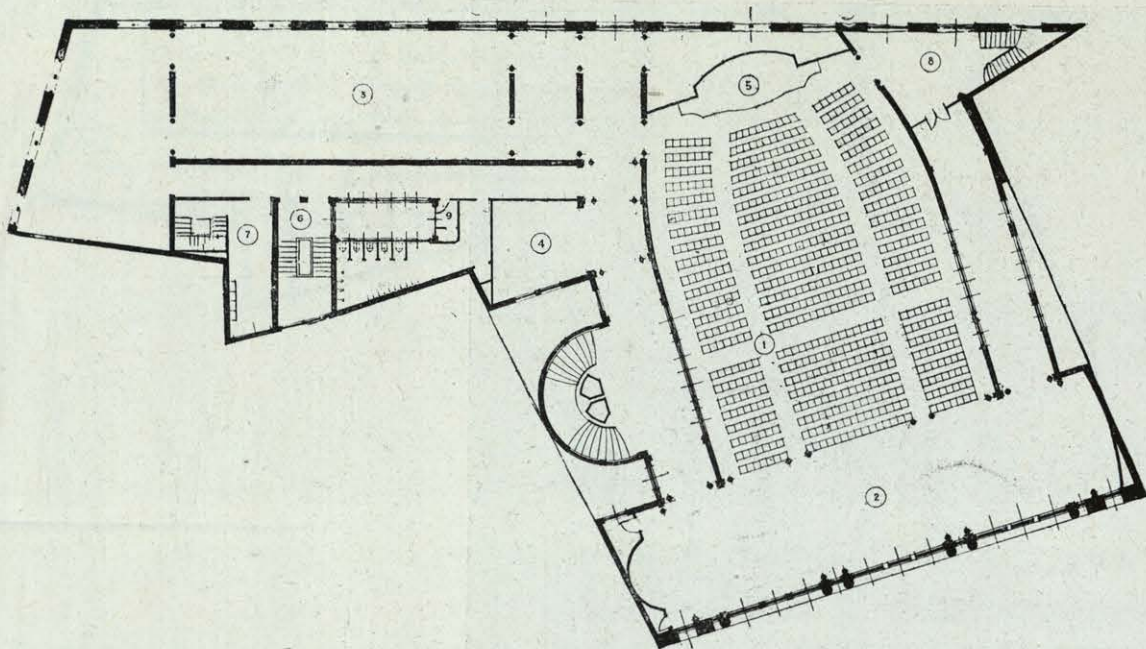
PLANTA TERCERA.—SOLUCIÓN D.
