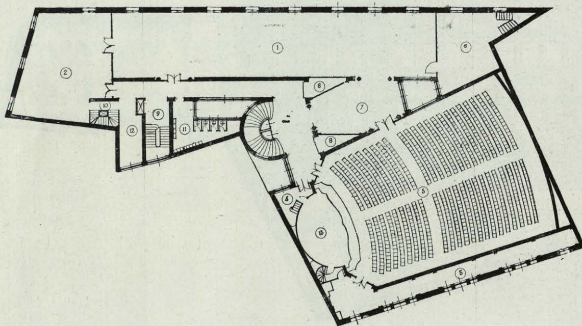
PLANTA SEGUNDA.—SOLUCIÓN A.
