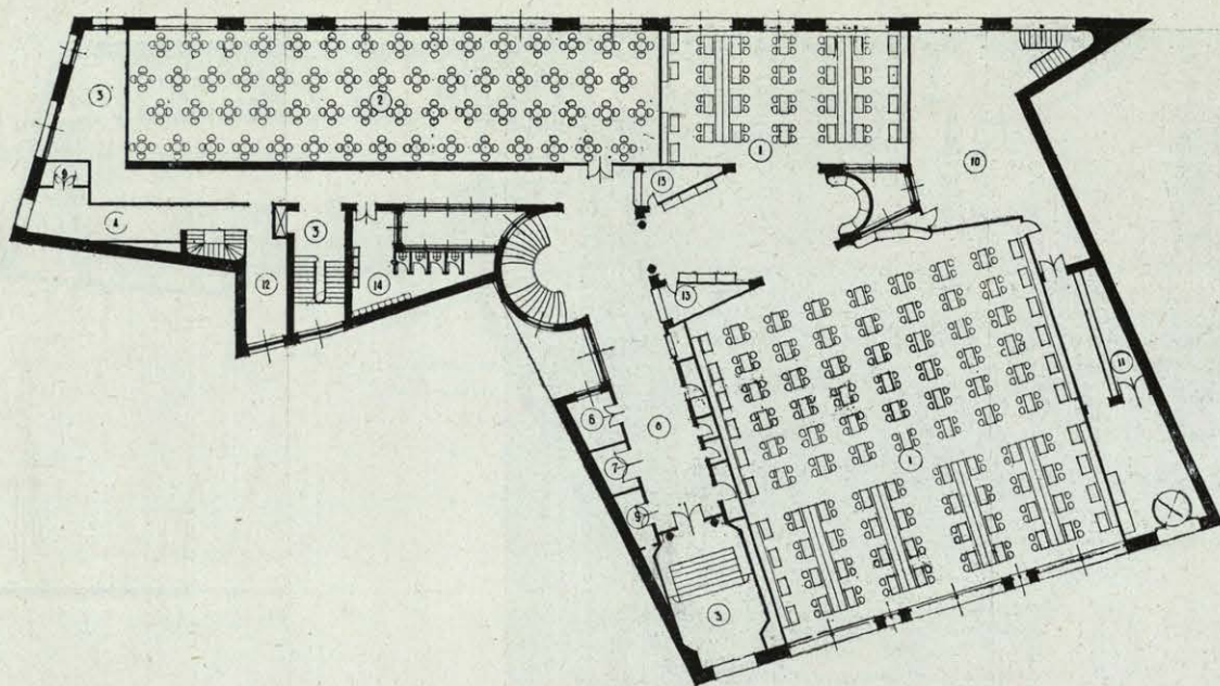
PLANTA BAJA.—SOLUCIÓN A.
